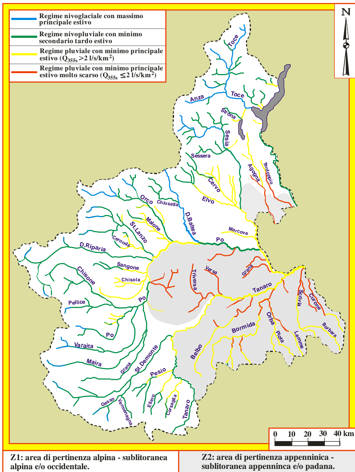
Fig. 17 - Classificazione dei regimi idrologici dei principali corsi d'acqua del reticolo idrografico piemontese e individuazione delle macro-tipologie Z1 (in chiaro) e Z2 (in grigio). Tutti le tipologie fluviali comprese nei parchi regionali impegnati nel progetto Interreg "Aqua" sono comprese nell'area Z1.
