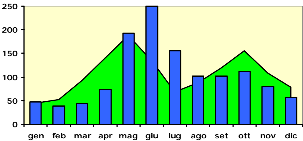
Fig. 6c - Regime idrologico dei valori medi mensili [mm] degli afflussi (A - area verde) e dei deflussi (D - istogrammi azzurri) a Crissolo - Nivoglaciale (103101).
