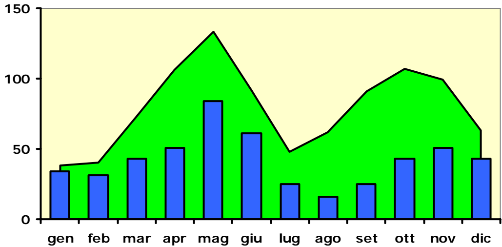
Fig. 6a - Regime idrologico dei valori medi mensili [mm] degli afflussi (A - area verde) e dei deflussi (D - istogrammi azzurri) a Moncalieri - Pluviale (103311).
