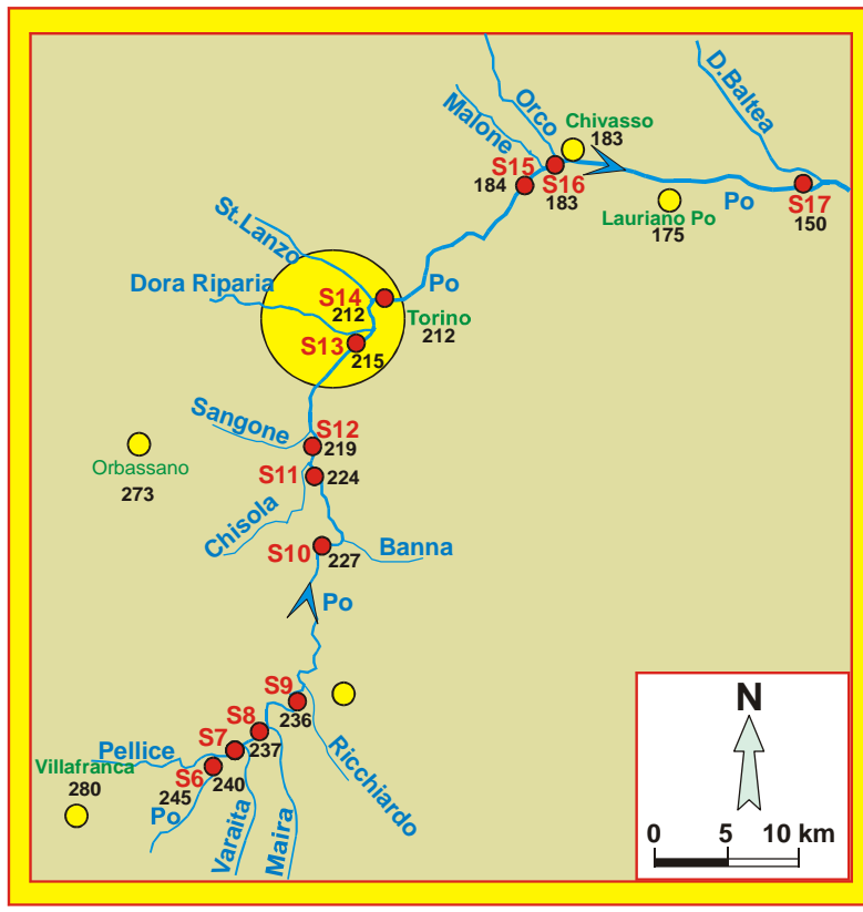
Fig. 3 - In alto è rappresentato il bacino dell'alto Po , (nel territorio cuneese) con la sua vetta più elevata (M.te Viso) a 3.841 m s.l.m. La sezione di chiusura è la S6 (245 m s.l.m.) presso Villafranca. La stessa sezione di riferimento è rappresentata anche in basso a sinistra della figura a lato. Verso valle sono indicate le altre sezioni lungo l'asta fluviale del Po in Provincia di Torino, fino alla S17 , a monte della confluenza con la Dora Baltea.
