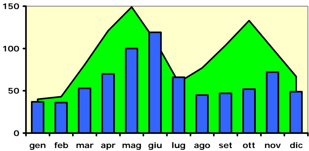
Fig. 6b - Regime idrologico dei valori medi mensili [mm] degli afflussi (A - area verde) e dei deflussi (D - istogrammi azzurri) a Cardè - Nivopluviale (103201).
