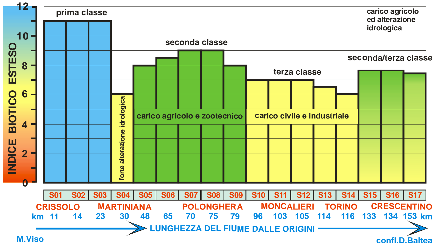
Fig. 16 - Qualità biologica delle acque valutata con la metodologia dell'Indice Biotico Esteso (IBE) valutata alle sezioni di riferimento 01 + 17 considerate sul tratto dell'asta fluviale del Po nei territori delle Province di Cuneo e di Torino.
