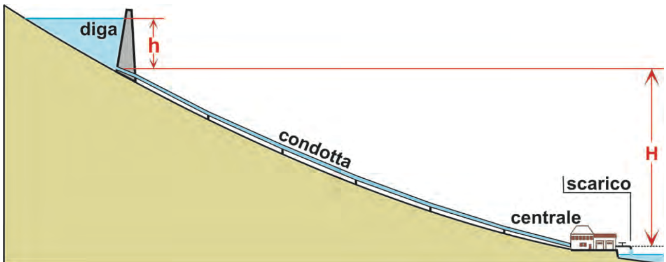
Fig. 2 - Una Centrale idroelettrica alimentata da una diga sfrutta il salto dato dalla somma del livello "h" del bacino artificiale e del dislivello altimetrico "H".
